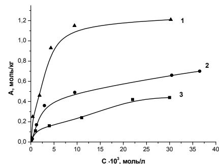
1 – хлопковая целлюлоза; 2 – МКЦ; 3 – МКЦ, модифицированная хитозаном Рис. 2 – Изотермы сорбции ионов меди из водных растворов
