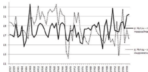
Рис.3. Максимальные температуры (подекадно) р. Нугуш (составлено автором).
