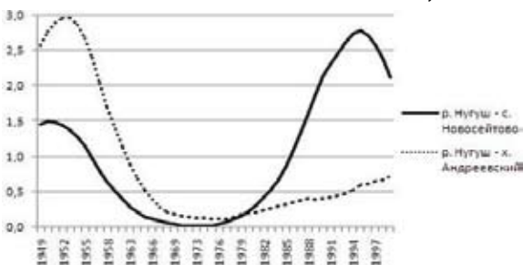
Рис.2. Динамика термического режима р. Нугуш (составлено автором методом 10-летних скользящих)
