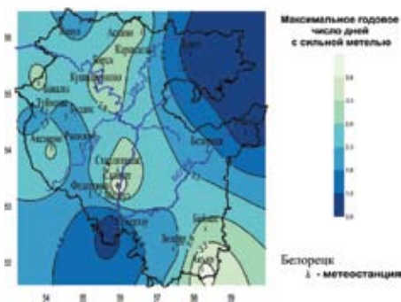
Рисунок 1. Максимальное число дней с сильной метелью на территории Республики Башкортостана (составлено автором по данным [1, 3])
