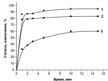
1 – хлопковая целлюлоза; 2 – МКЦ; 3 – МКЦ, модифицированная хитозаном Рис. 1 – Кинетические кривые сорбции ионов меди из водных растворов
