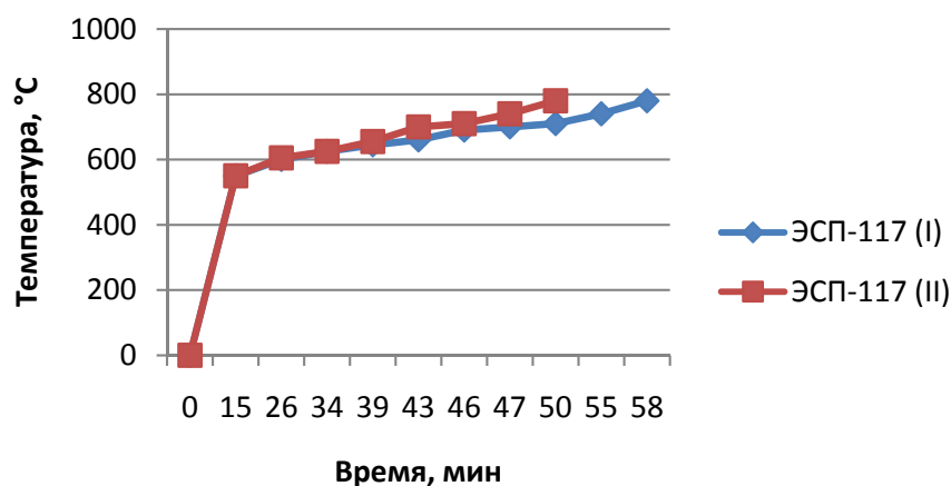
Рисунок 1 – График плавкости стеклоэмалей ЭСП-117 (I) и ЭСП-117 (II)
